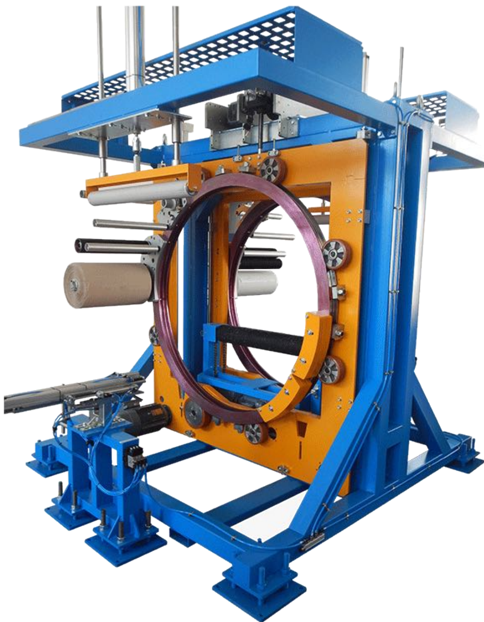
Автоматичний обмотувач RING 100
